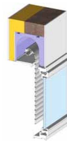
Coffre Tunnel avec isolation par l'extérieur
